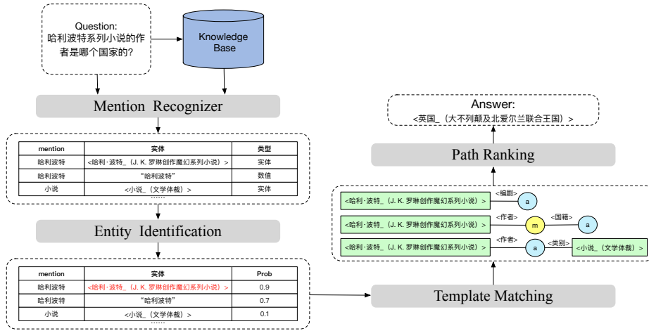
图 1. 系统整体流程图, 本系统包括指称识别、实体链接、模板匹配和路径排序四个组件。
